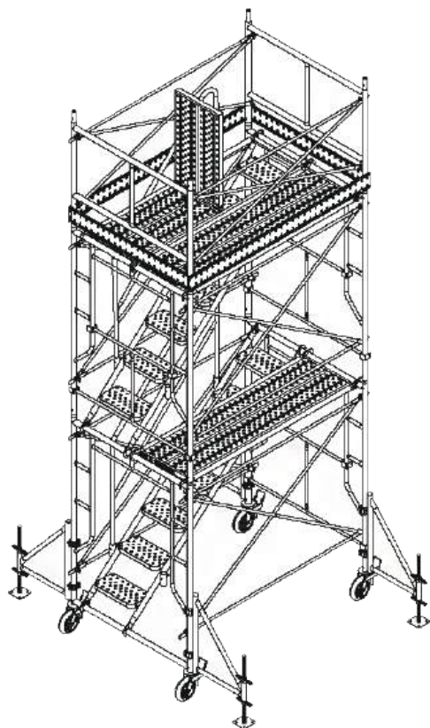
▲ CN4750上下設備(施工架)
