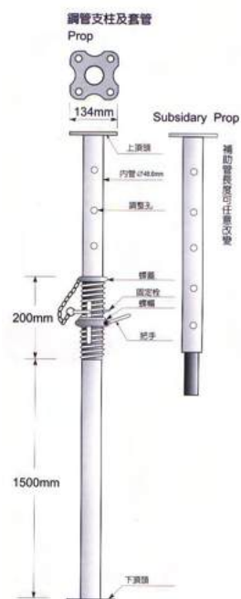
▲ 支撐鋼管
